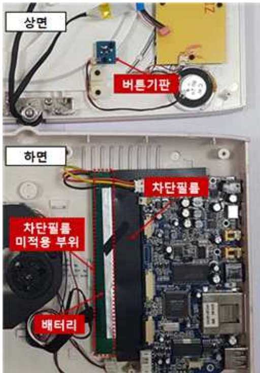
<제품 내부구조>
